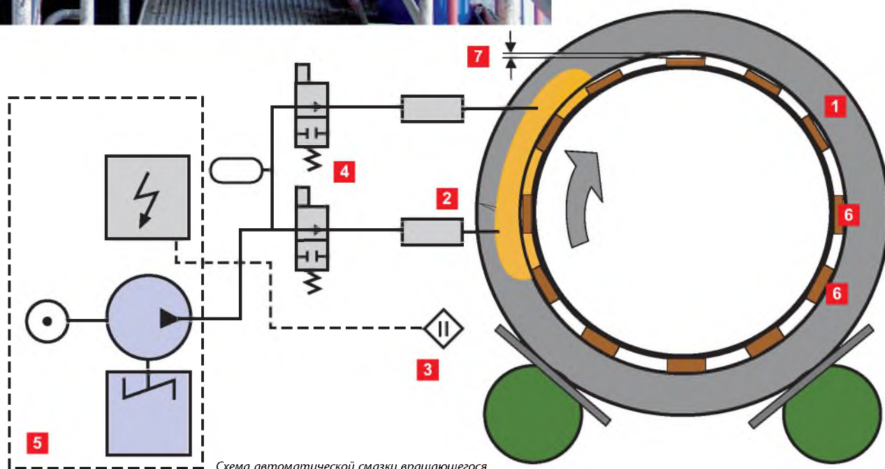
Схема автоматической смазки вращающегося кольца
